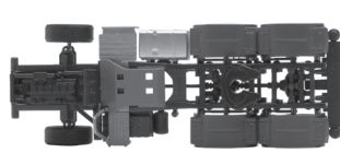
085328 H0 1:87 Fahrgestell Zugmaschine 3achs MAN TGX/TGS 6x4 mit Heckabstützung und Konsole für Ladekran (2 Stück) / chassis MAN 6x4 with rear support and console for loading crane (2 pieces)
